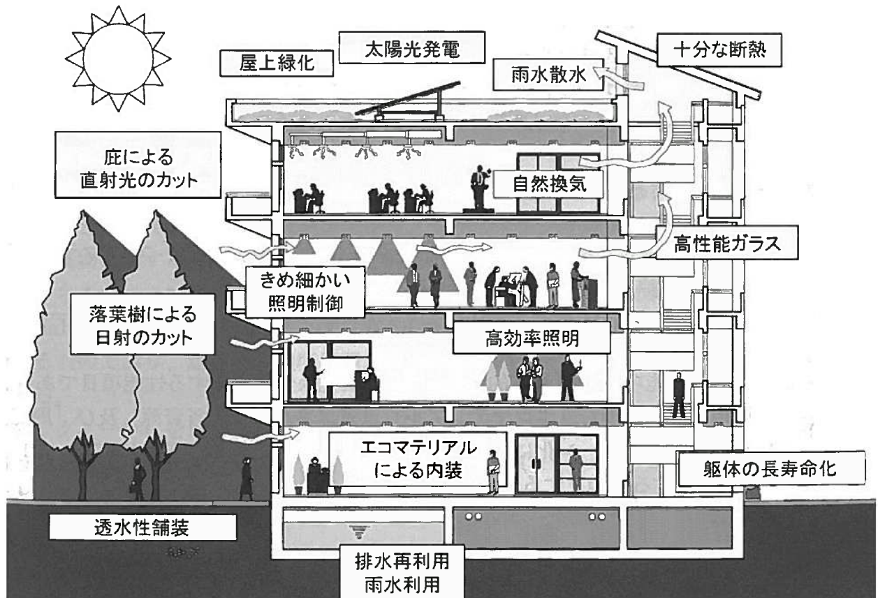
図 7-19 環境配慮型庁舎のイメージ [国土交通省 グリーン庁舎基準及び同解説]
