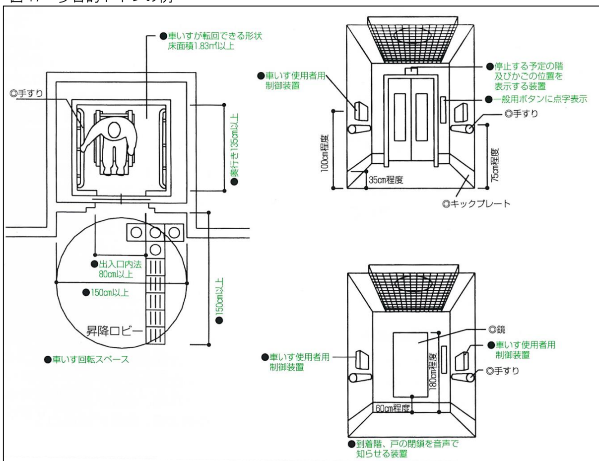
図 18 エレベーターの整備例[鹿児島県福祉のまちづくり条例施設整備マニュアル]
