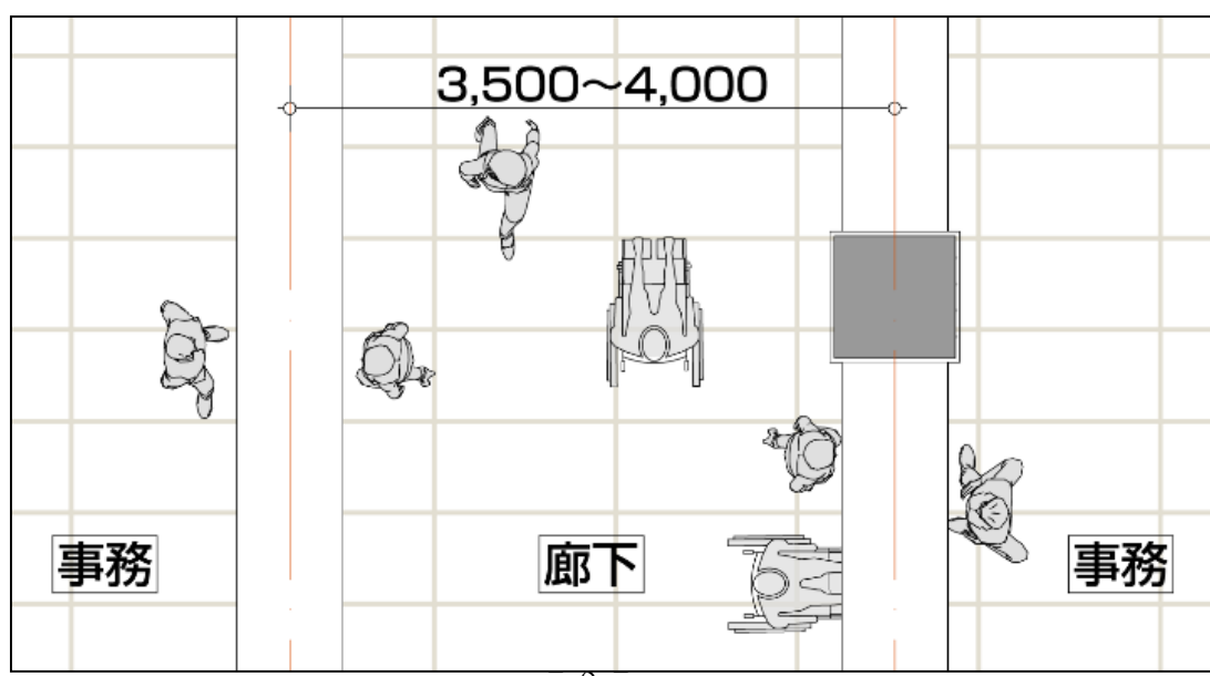
図 16 ゆとりのある廊下幅の例
