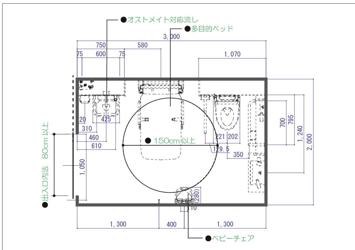
図 17 多目的トイレの例
