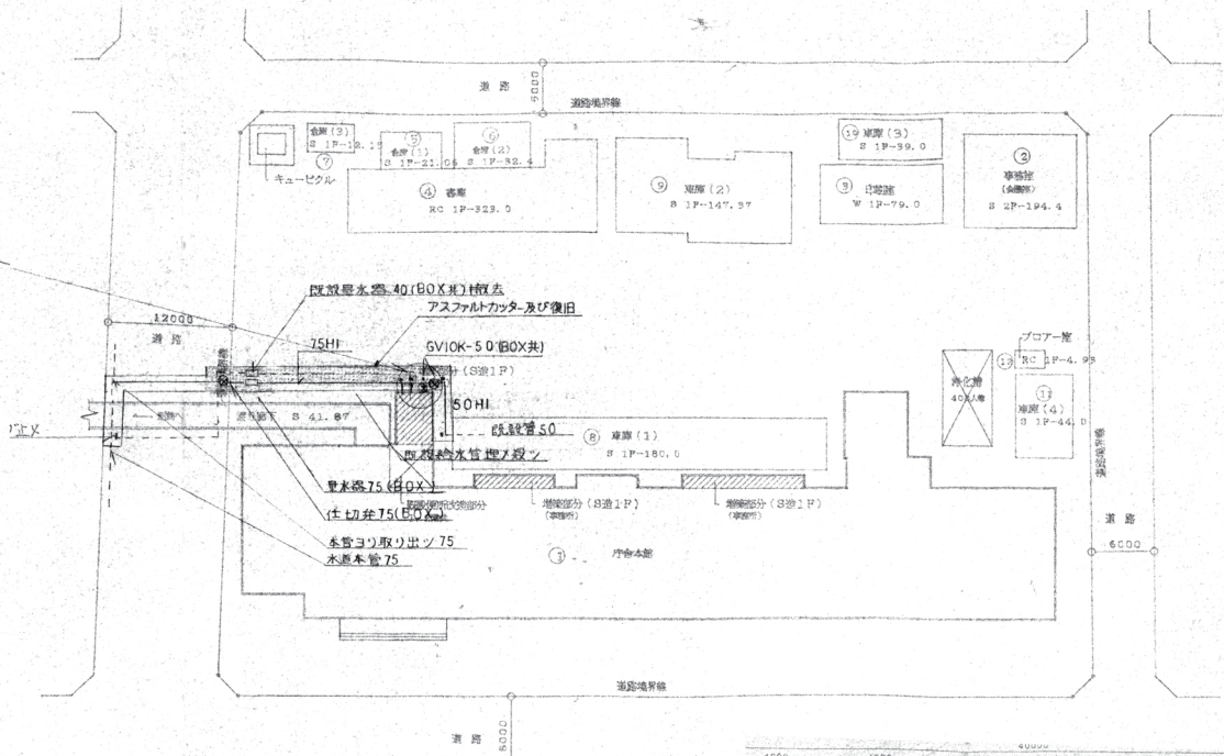
配管図 1:400
