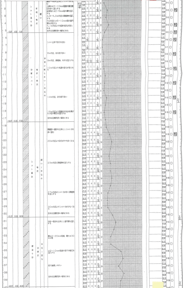
参考資料 6-3 2号館ボーリング柱状図 (No.1)
