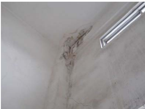
図 2-11 防水層の劣化と躯体のひび割れによる漏水痕（加治木庁舎）
