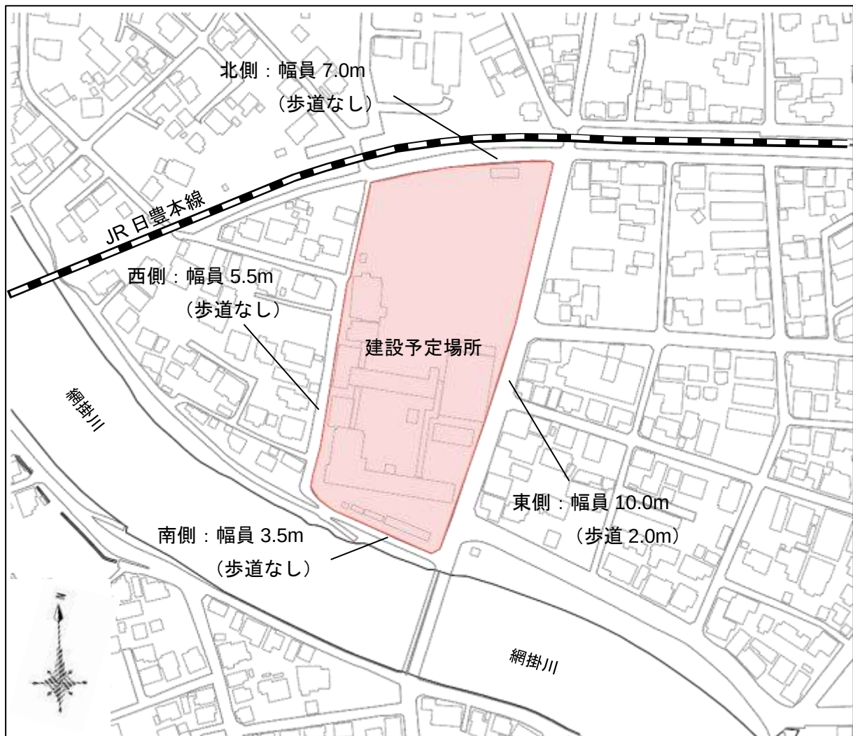
図 3-2 総合支所庁舎周辺の道路状況
