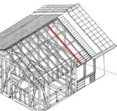
垂木（たるき）
